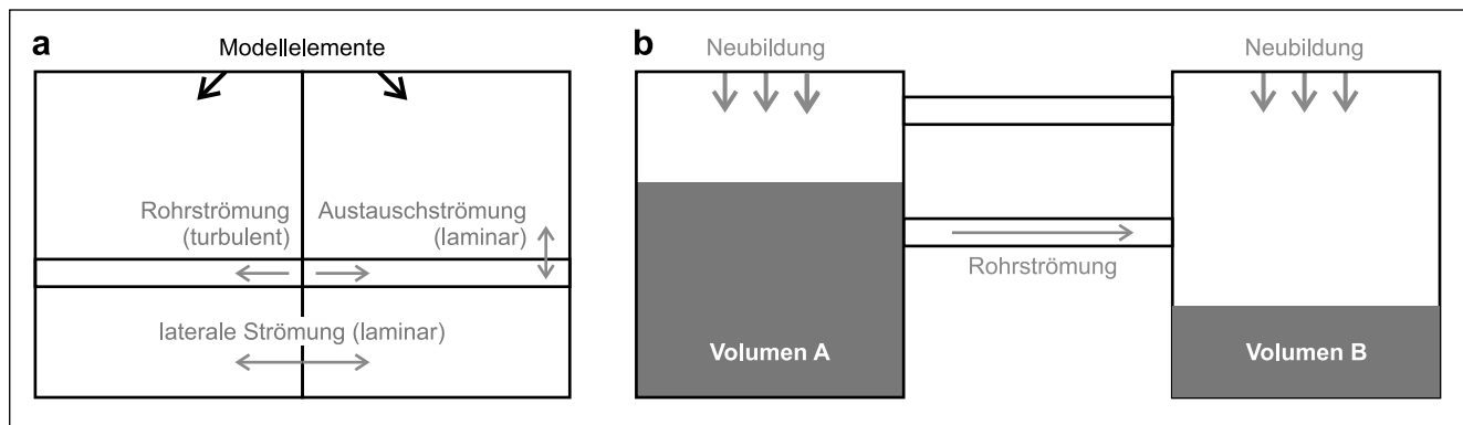
Abb. 1 Konzeptionelle Modellvorstellung von (a) einem diskreten Hohlraummodell und (b) einem Parametermodell wie dem Box Modell. In einem diskretisierten Kontinuummodell werden die Strömungstypen vergleichbar dem Hohlraummodell (a) implementiert
